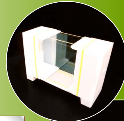
ソーラーセル搬送Lパッドタイプ
